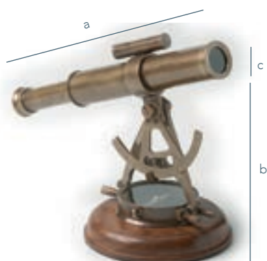
333 012 TEODOLITO/THEODOLITE a : 22,2 cm b : 18,5 cm c : Ø 3,3 cm Pie/Pied/Stand Ø 12 cm
